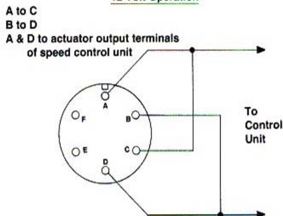
DIAGRAM 5 12 Volt Operation
