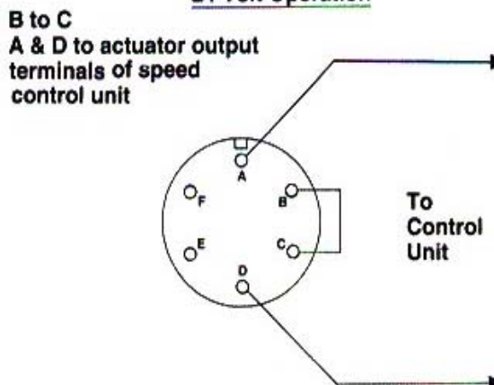
DIAGRAM 6 24 Volt Operation
